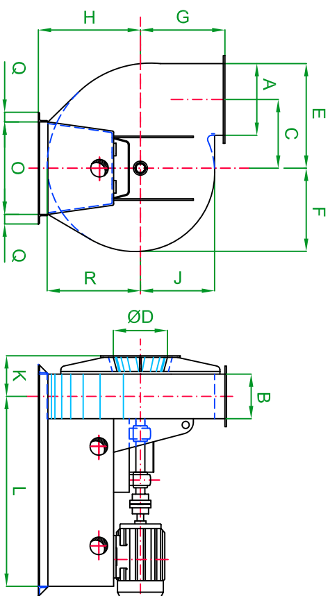
K 35 - Bauart Grundtype - Ø Saugöffnung / Totaldruckhöhung - Volumenstrom
