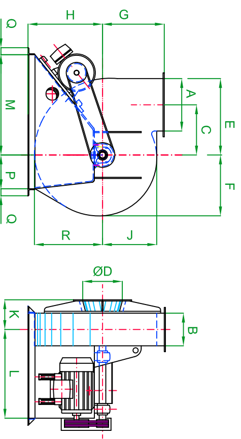
R 35 - Bauart Grundtype - Ø Saugöffnung / Totaldruckhöhung - Volumenstrom
