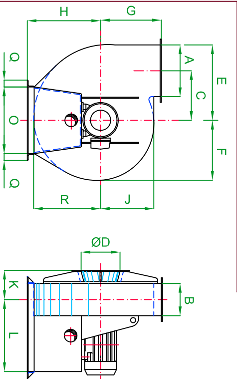
M 35 - Bauart Grundtype - Ø Saugöffnung / Totaldruckhöhung - Volumenstrom
